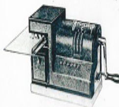
Francotyp C
